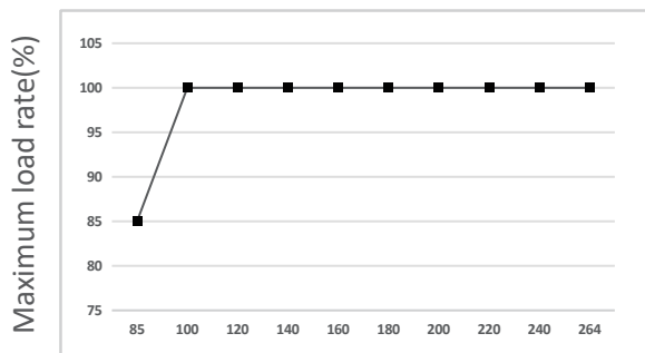
Input Voltage(Vac)
