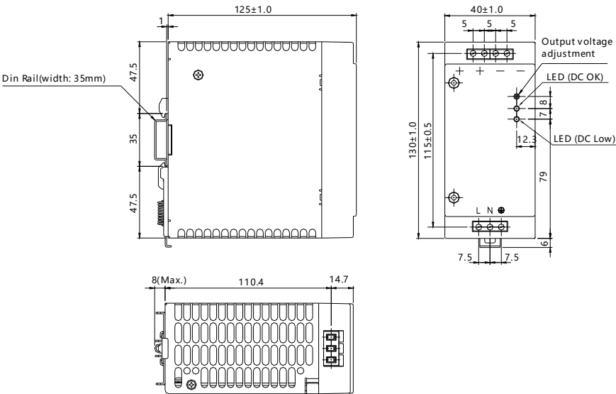
Unit:mm Tolerance:±1.0
